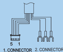
CONNECTOR : MOLEX 5264-05 (SBDM-10A)
