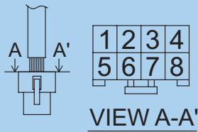
CONNECTOR : MOLEX 5557-08 (SBDM-05A)
