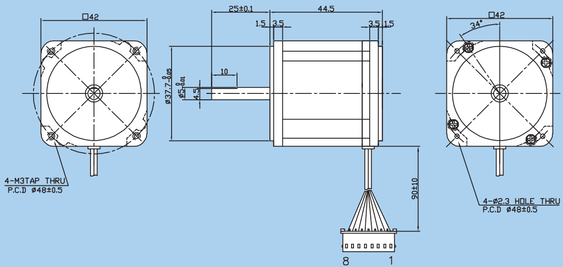
CONNECTOR(CHB0640-8)
